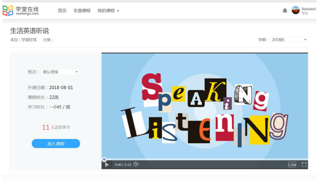
图 2.6 课程介绍页
