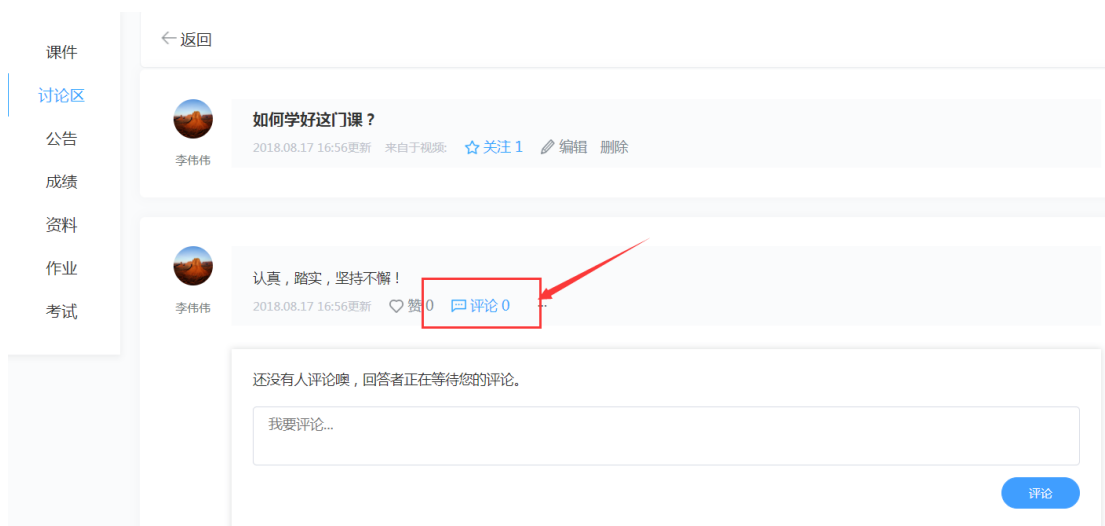
图 3.9 评论和点赞
