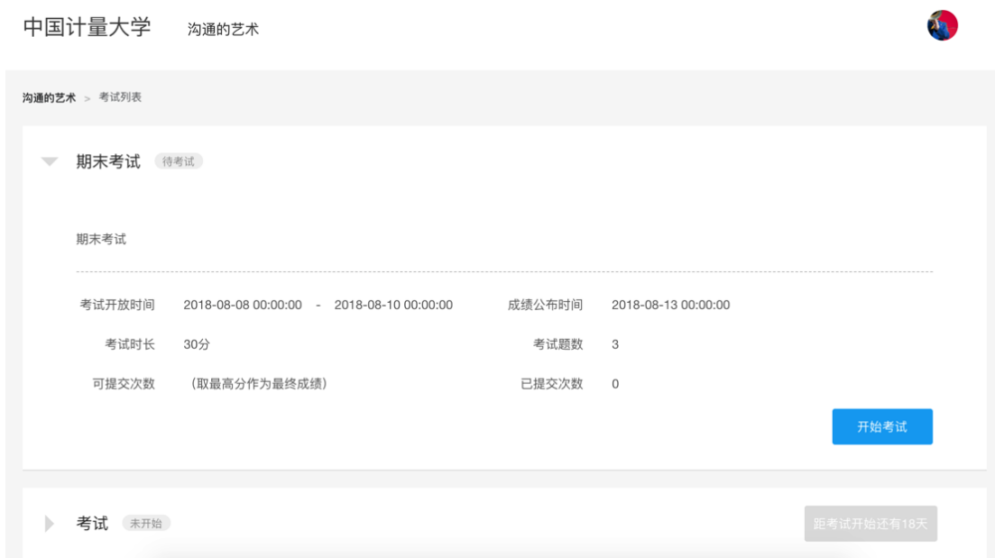
图 3.22 考试入口
