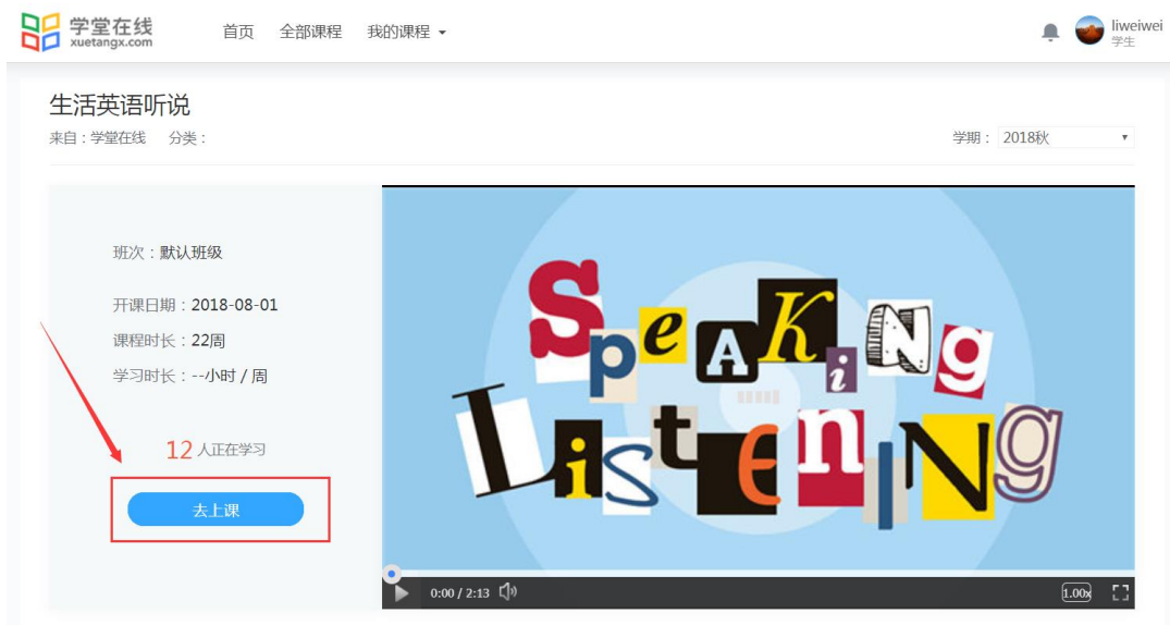
图 2.7 去上课页面
