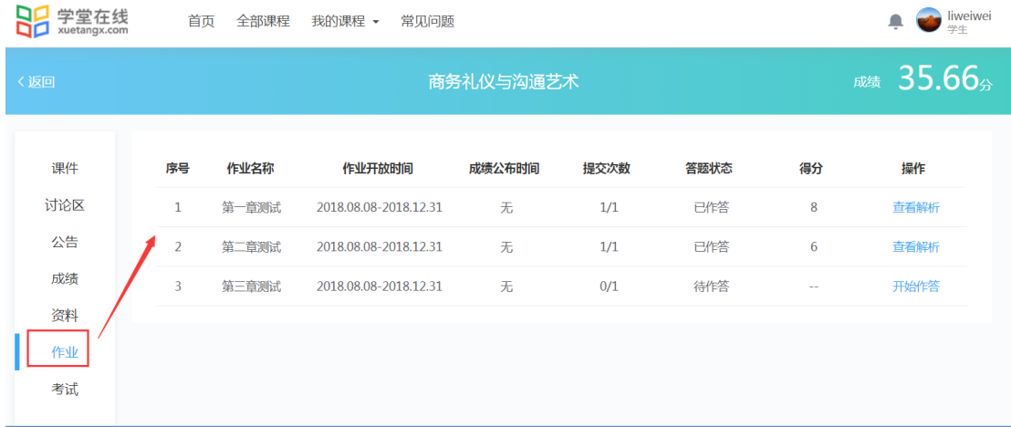
图 3.20 作业入口 2
